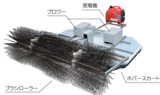
＜秋田式水田ロボット除草機＞
